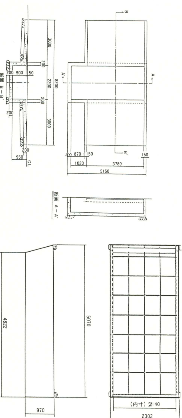
コンクリート製ビット (作業所施工)
